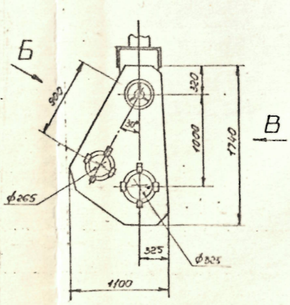
I Н 1:20 подвеска 180 т
