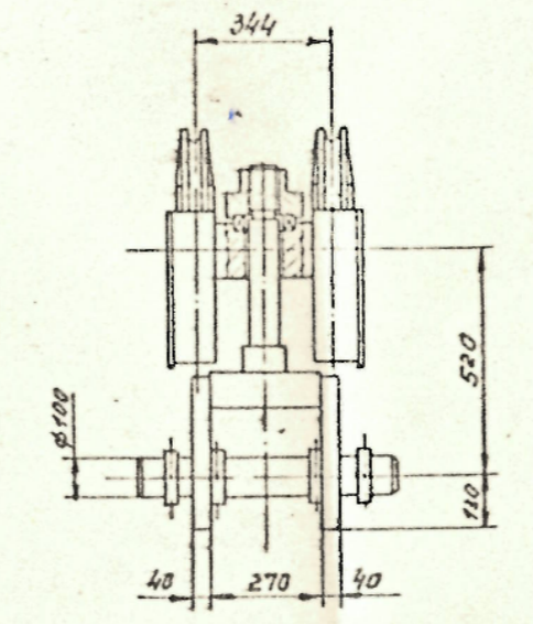
II вариант Н 1:10 При маневрировании с затворами (шифры 283 РР) и решетками (шифры 284 РР)
