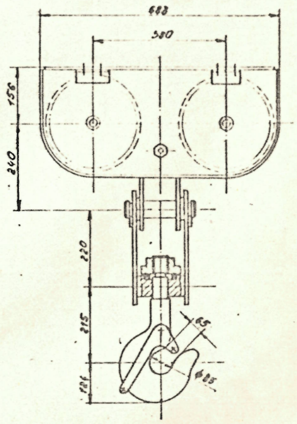
VI Н 1:5 подвеска 5 т
