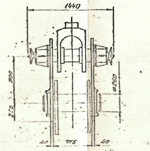
Вид Б варианты Н 1:20 При работе с затворами диаметром (шифры 213 РР, 401 Р)
