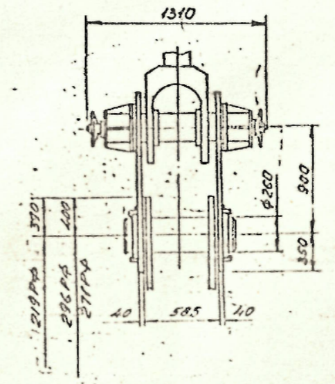
При маневрировании с затворами (шифры 219 РР, 296 РР, 271 РР)
