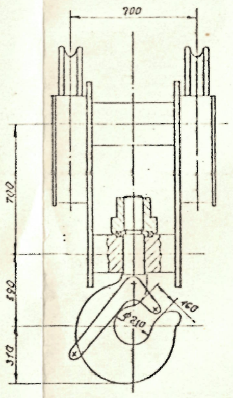
III Н 1:10 подвеска 40 т
