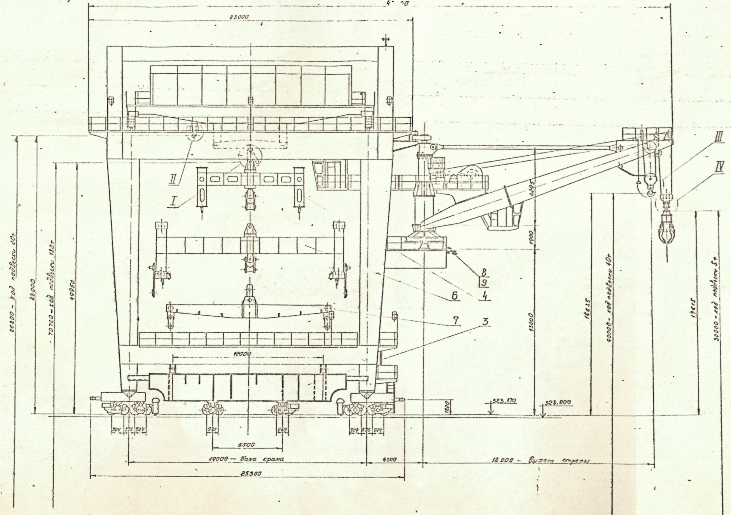
Вид А лист 1. (стрела развернута в плоскости чертежа на 90°) Н 1:75
