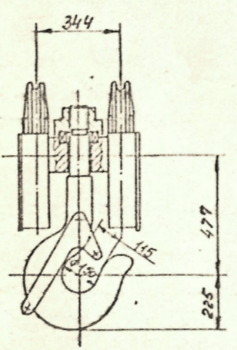
II Н 1:10 подвеска 20 т
