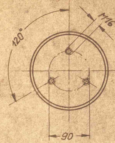
Ansicht in Richtung Bug по стрелке "X" M 1:5
