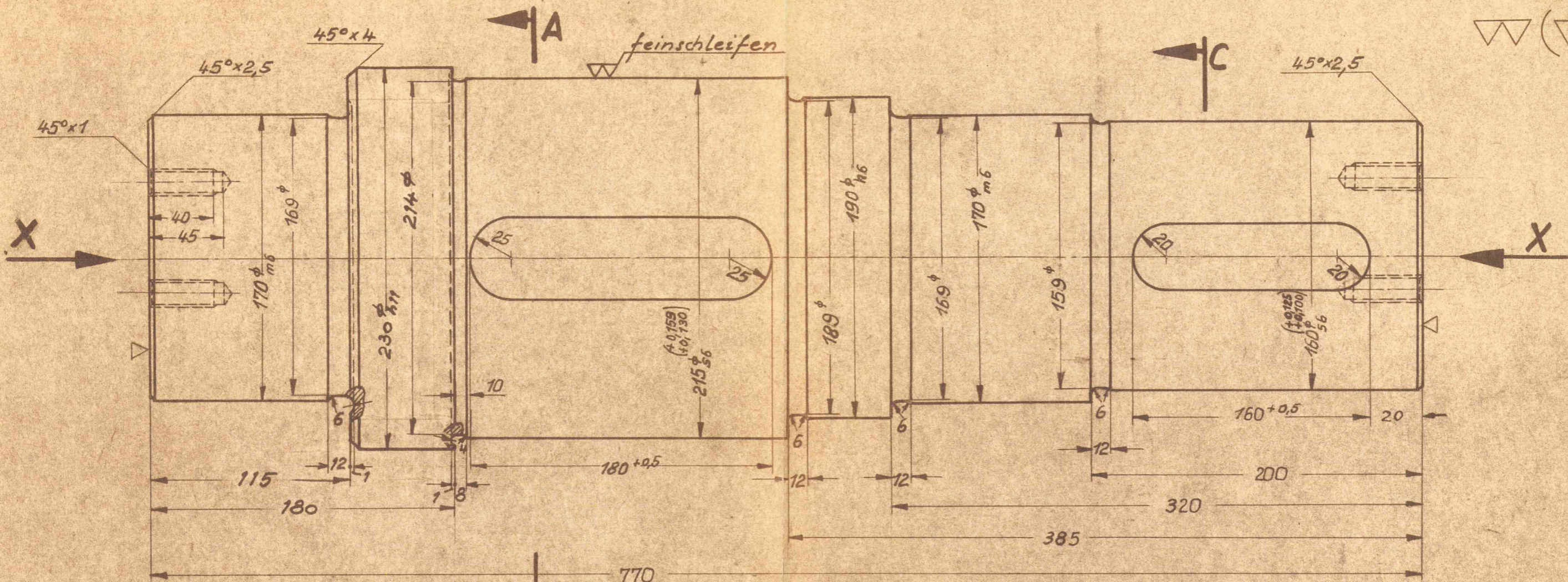
Ansicht in Richtung Bug по стрелке "X" M 1:5
