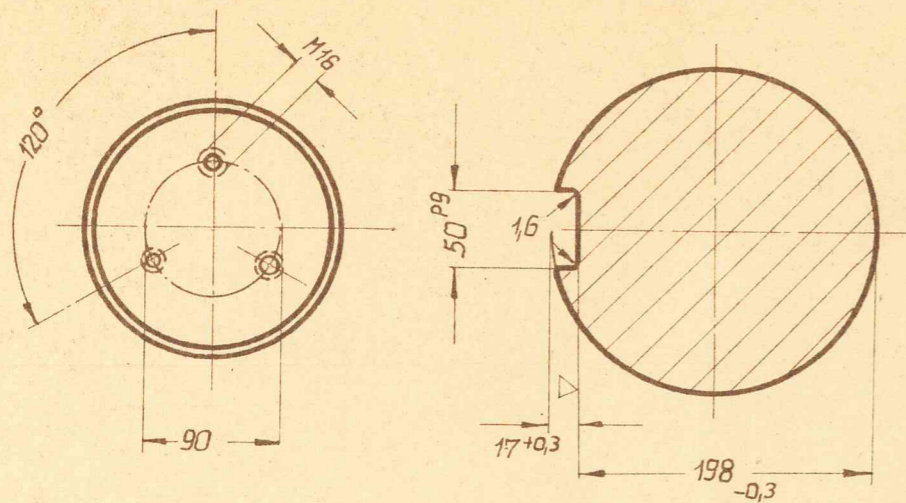
Schnitt Разрез A-B M 1:1
