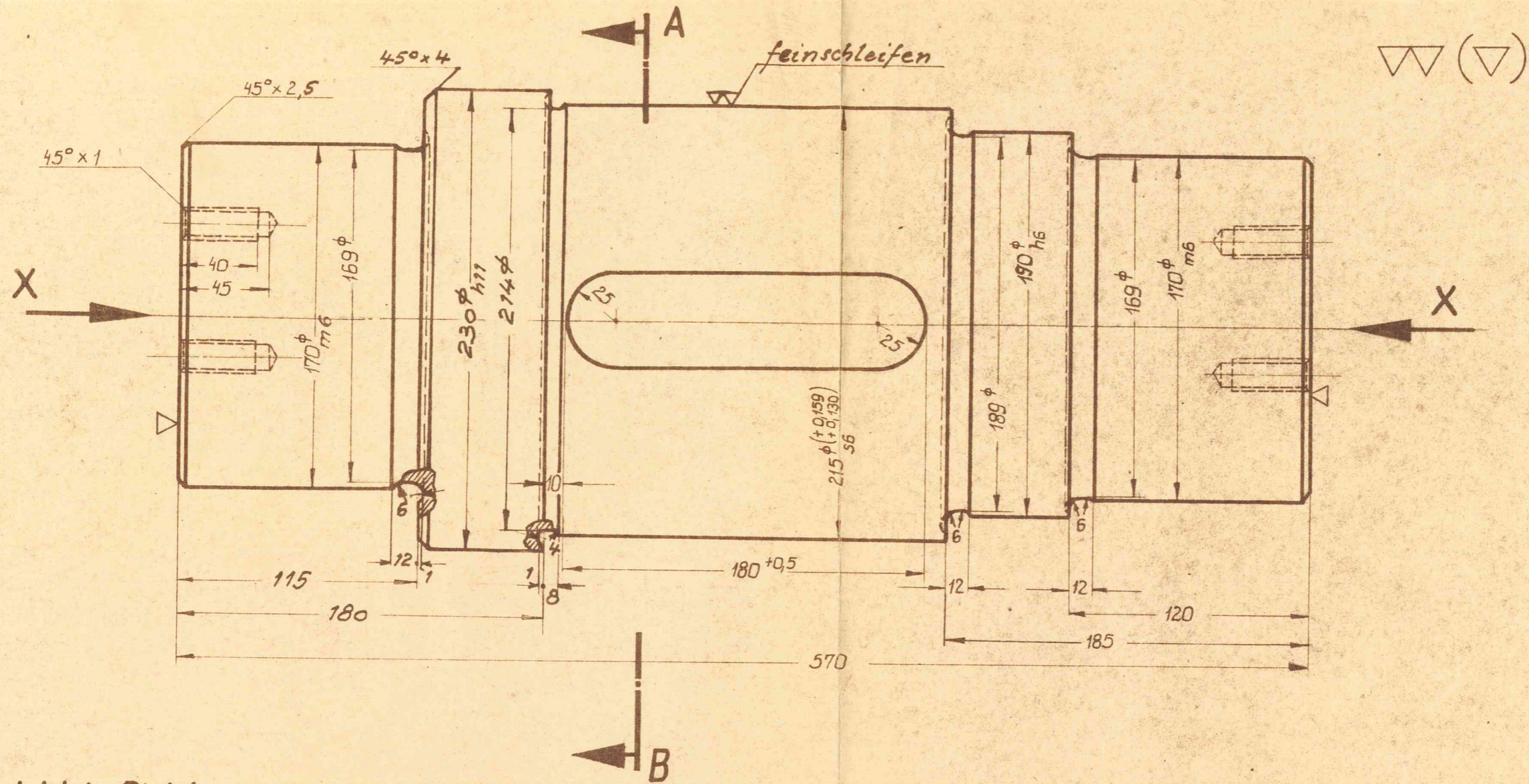
Schnitt Разрез A-B M 1:1
