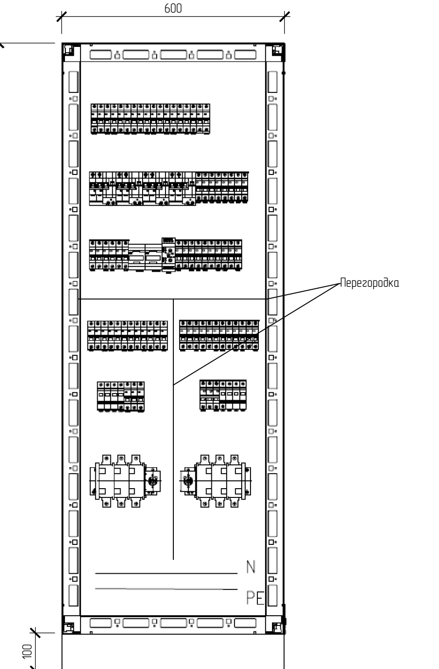
Общий вид шкафа ШРСБ3
