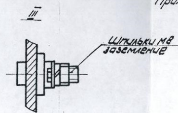
Вид Е Крышка условно не показано
