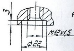
Г-Г Пробка и прокладка условно не показаны
