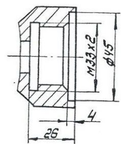
I повернуто Пробка и прокладка условно не показаны
